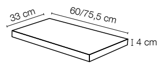
Angolare (assemblato)
